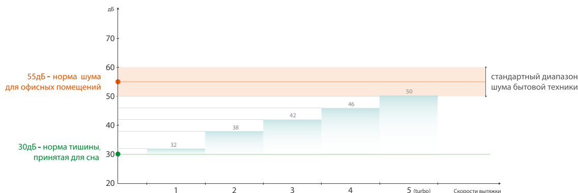
Диаграмма уровня шума на пяти скоростях работы вытяжки KRONAsteel AIDA Silent.
